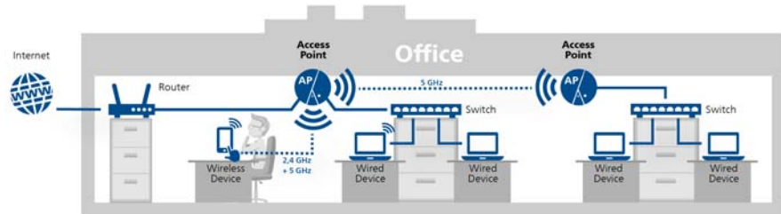
Abb. 3: WDS-Bridge
