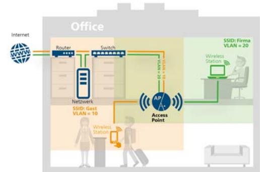
Abb. 4: Statisches VLAN
