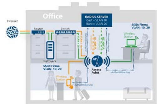
Abb. 5: Dynamisches VLAN
